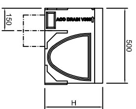
Latakas L-0,5 m su rūsiniu vamzdzim Ø200; su rūsiniu "L", "T" formos linijai formuoti
