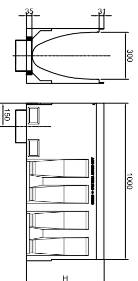
Latakas L-1,0 m su anga ir tarpine vamzdzim Ø200
