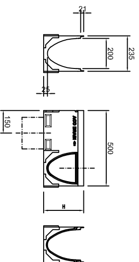
Latakas L-0,5 m su ruošiniu vamzdiu Ø200; su ruošiniu "L", "T" formos linijai formuoti
