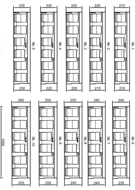
Latakas L-1m, su dugno nuolydziu f=0,5%
