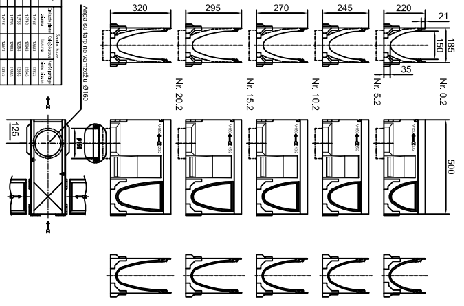
Latakas L-0,5 m su su anga r tarpine varanzdziu Ø160, su ruosiniu T 1 , T 2 formos Inijiai formuoti
