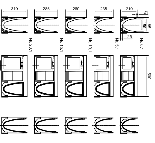
Roostine su anga Ø160
