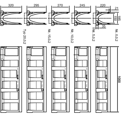
Latakas L-1m su anga r tarpine varanzdziu Ø160
