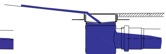
Montavimas ties įėjimu (vandens patvanka nepageidaujama)
