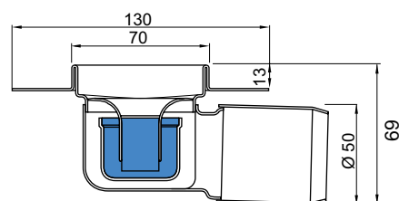
Sekliojo latakų matmenys (statybinis aukštis 69 mm)
