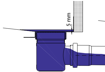
Montavimas ties siena (vandens patvanka iki 5 mm)
