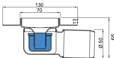
Seklijo latakų matmenys (statybinis aukštis 65 mm)
