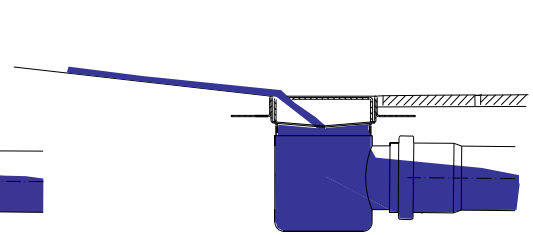
Montavimas ties jėjimu (vandens patvanka nepageidaujama)
