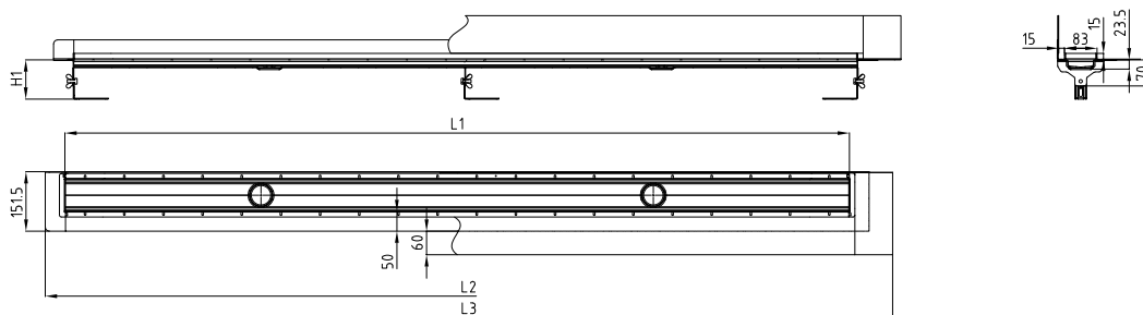
Latakas su vertikalia sandarinimo jungė (flanšu)
