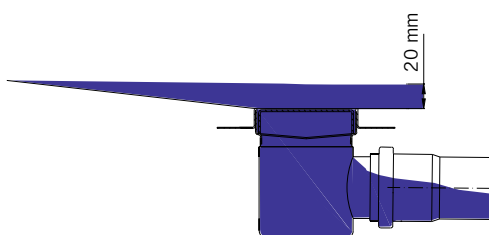
Pralaidumo testas pagal EN 1253-1
