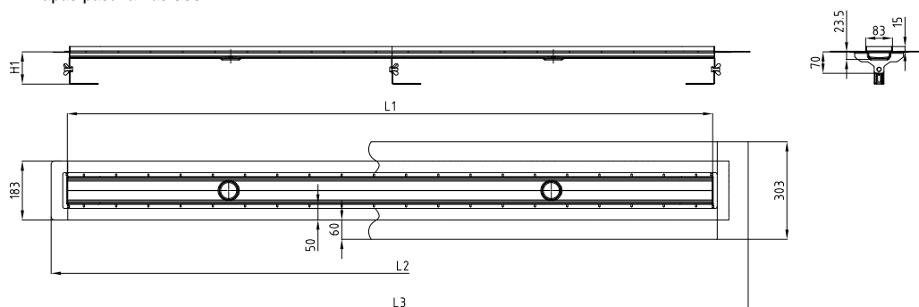
Latakas su horizontalia sandarinimo jungė (flanšu)
