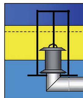
Maksimalus lengvųjų skysčių kiekis Ištekėjimas automatiškai uždaromas plūdiniu mechanizmu
