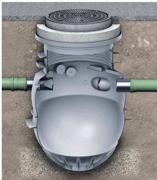
Montavimo pavyzdyje pavaizduota ACO Pitumax P 750 su B 125 apkrovos klasės viršutine dalimi.
