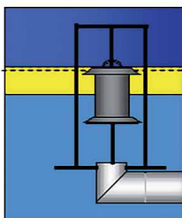
Darbinis režimas Lengvųjų skysčių kaupimasis
