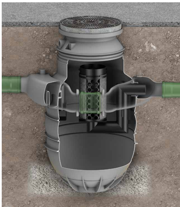
Montavimo pavyzdyje pavaizduotas ACO Oleopass P-SD NS 3 su B 125 apkrovų klasės viršutine dalimi.
