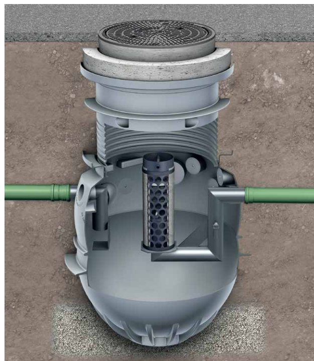
Montavimo pavyzdyje pavaizduotas ACO Oleopator P NS 3 su B 125 apkrovos klasės viršutine dalimi.
